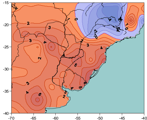
Figura 1: Tendencia de la precipitación anual en mm/año. Período 1960-2000
