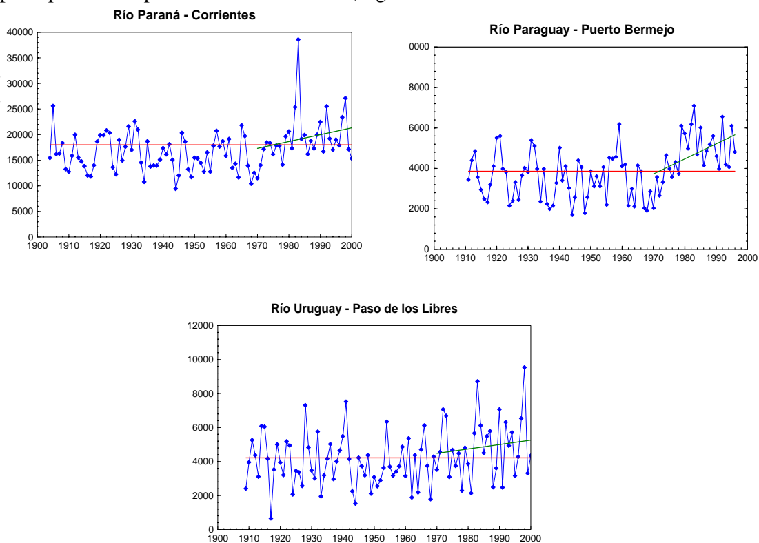
Figura 4: Caudales medios anuales ( m^3/s ) en los ríos Paraná, Paraguay y Uruguay. Promedios para el período (línea roja) y tendencia lineal a partir de 1970 (línea verde)
