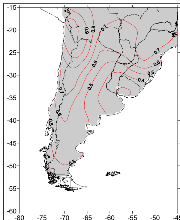
Figura 11: Cambio de temperatura media anual (° C) para el período 2020-40 respecto de 1991-2000 para el escenario A1b derivado de un ensamble de 14 MCGs (Versión 2006) Las áreas sombreadas son significativas al 5%. Gentileza de I. Camilloni
