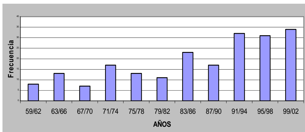
Figura 3: Precipitaciones mayores a 100 mm en no más de dos días en 16 estaciones de la región Centro y Este de Argentina. Las frecuencias muestran el número de casos en los periodos de cuatro años indicados
