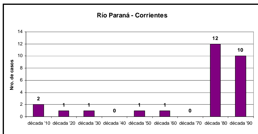
Figura 5: Frecuencia decádica de casos en los que el caudal mensual supera en al menos dos veces el desvío estándar para el correspondiente mes.
