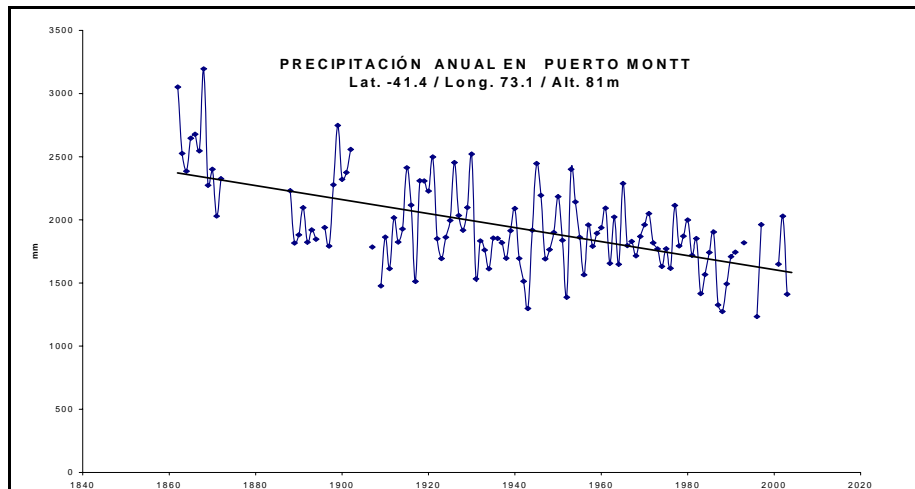
Figura 7: Precipitación media anual y tendencia lineal. Puerto Montt (arriba) y La Serena (abajo)
