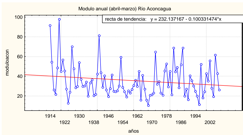
Figura 8: Caudales medios anuales ( m^3/s ) en el río Aconcagua. Se indica la tendencia lineal para el período total con información disponible (línea roja)
