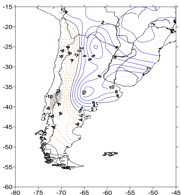
Figura 10: Cambio de precipitación media anual (%) para el período 2020-40 respecto de 1991-2000 para el escenario Alb derivado de un ensamble de 14 MCGs (Versión 2006) Las áreas sombreadas son significativas al 5%. Gentileza de I. Camilloni
